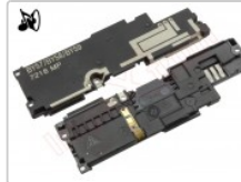
Módulo de antena con altavoz tono de llamada para sony xperia xa1, g3121
